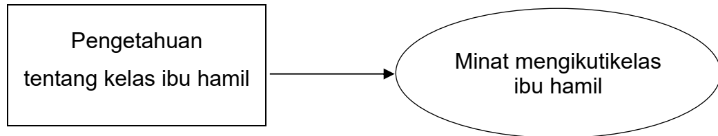
Gambar 3.1 Kerangka Konseptual
